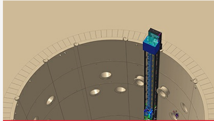
CEA Cadarache : Réacteur Jules Horowitz (RJH) - Dispositif expérimental ADELINÉ
